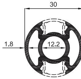
M1-10/A (4,6 Kg / 6 mt) 30 mm İki Kanallı Dikme 30 x 1.8 mm Strut With Two Channel Poteau rond 30x1,8 mm double rainures دعامة أو بروفيل دائري بقتاتين 30x1.8 MM
