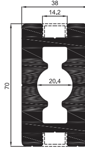
MK-06/HD (29,4 Kg / 6 mt) 70 x 38 Dikdörtgen Çift Kanallı Dikme Hd 70 x 38 Rectangular Two Channelled Strut Hd Poteau rectangulaire Plein 70x38 mm double rainures دعامة أو بروفيل مدعم مستطيل ذو قناتين 70x38 HD
