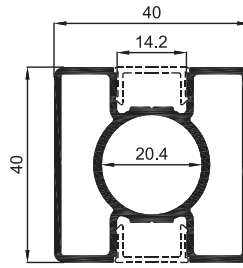
MK-07 (6,1 Kg / 6 mt) 40 x 40 Kare Çift Kanallı Dikme 40 x 40 Square Two Channelled Strut Poteau carré 40x40 mm double rainure دعامة أو بروفيل مدعم مربع ذو قناتين 40x40
