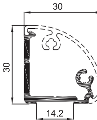
ME-07 (2,5 Kg / 6 mt) 30 x 30 Elips Panel Profili 30 x 30 Ellipse Panel Profile ( Channel 14,2 Mm ) Profil ovale 30x30 mm بروفيل قاعدي بيضوي 30x30 (14.2 MM)
