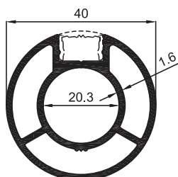
M1-04/B (5,65 Kg / 6 mt) 40'lık Dikme Tek Kanallı 40 x 1.6 mm Strut With One Channel Poteau rond 40x1,6 mm une rainure دعامة أو بروفيل دائري بفتاة واحدة 40x1.6 MM
