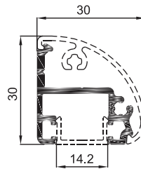
ME-06 (2,6 Kg / 6 mt) 30 x 30 Elips Etek Cam Profil 30 x 30 Ellipse Bottom Profile ( Channel 14,2 mm ) Support verre ovale 30x30 mm بروفيل قاعدي بيضوي للزجاج 30x30 (14.2 MM)
