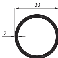
M1-03/A (3 Kg / 6 mt) 30 x 2 mm Alüminyum Boru 30 x 2 mm Aluminium Pipe Tube rond Aluminium 30x2 mm أنبوب الألمنيوم دائري 30x2 MM
