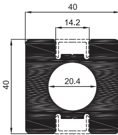
MK-07/HD (17,5 Kg / 6 mt) 40 x 40 Kare Çift Kanallı Dikme Hd 40 x 40 Square Two Channelled Strut Hd Poteau carré Plein 40x40 mm double rainure دعامة أو بروفيل مدعم مربع ذو قناتين 40x40 HD
