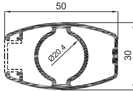
ME-05 (5,6 Kg / 6 mt) 50 x 30 Elips Tek Kanallı Dikme 50 x 30 Ellipse One Channeled Strut Poteau ovale 50x30 mm une rainure دعامة أو بروفيل بيضوي ذو قناة واحدة 50x30
