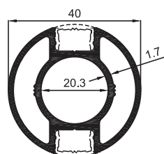
M1-04/A (5,4 Kg / 6 mt) 40'lık Dikme İnce 40 x 1.7 mm Strut With Two Channel Poteau rond 40x1,7 mm double rainures دعامة أو بروفيل دائري بفتاتين 40x1.7 MM
