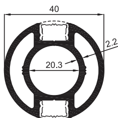
M1-04 (6,7 Kg / 6 mt) 40'lık Dikme Kalın 40 x 2.2 mm Strut With Two Channel Poteau rond 40x2,2 mm double rainures دعامة أو بروفيل دائري بفتاتين 40x2.2 MM
