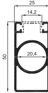
MK-06 (5,4 Kg / 6 mt) 50 x 25 Dikdörtgen Tek Kanallı Dikme 50 x 25 Rectangular One Channelled Strut Poteau rectangulaire 50x25 mm une rainure دعامة أو بروفيل مدعم مستطيل ذو قناة واحدة 50x25
