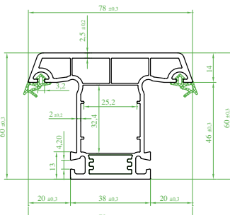
(ST 6122) "SÜPERTEC" Yeni Orta Kayıt Profili (Contalı) New Mullion Profile (Seal) Профиль импоста, новый (с уплотнителем) بروفیل المنصف الثابت جدید (مع القفیل)
