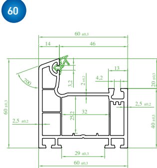
(ST 6111) "SÜPERTEC" Yeni Kasa Profili (Contalı) New Frame Profile (Seal) Профиль коробки, новый (с уплотнителем) بروفیل الصندوق جدید (مع قفیل)
