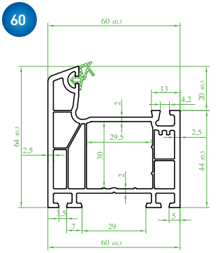
(ST 9110) "EXTRATEC" Kasa Profili (Contalı) Frame Profile (Seal) Профиль коробки (с уплотнителем) بروفیل الصندوق (مع قفیل)
