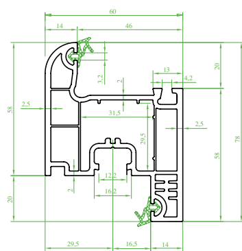
(ST 4310) "SOLOTEC" Kanat Profili (Contalı) Sash Profile (Seal) Профиль створки (с уплотнителем) بروفیل الضرفه (مع القفیل)
