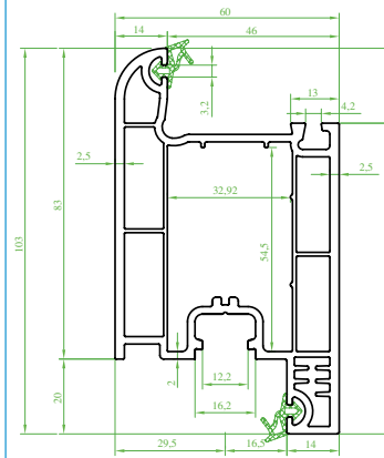
(ST 3410) "OVALTEC" Kapı Kanat Profili (Contalı) Door Sash Profile (Seal) Профиль дверного полотна (с уплотнителем) بروفیل ضرفه باب (مع القفیل)
