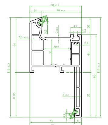
(ST 1410) "GROSSTEC" Pervazlı Kasa Profili (Contalı) Edge Frame Profile (Seal) Профиль коробки с карнизом (с уплотнителем) بروفیل الصندوق ذو البرواظ (مع القفیل)
