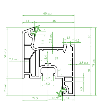
(ST 9310) "EXTRATEC" Kanat Profili (Contalı) Sash Profile (Seal) Профиль створки (с уплотнителем) بروفیل الضرفه (مع القفیل)
