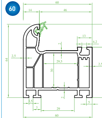
(ST 3110) "OVALTEC" Kasa Profili (Contalı) Frame Profile (Seal) Профиль коробки (с уплотнителем) بروفیل الصندوق (مع قفیل)
