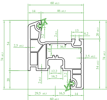
(ST 6133) "SÜPERTEC" Yeni Kanat Profili (Contalı) New Sash Profile (Seal) Профиль створки, новый (с уплотнителем) بروفیل الضرفه جدید (مع القفیل)
