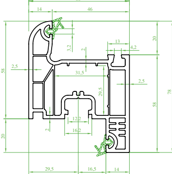
(ST 3310) "OVALTEC" Kanat Profili (Contalı) Sash Profile (Seal) Профиль створки (с уплотнителем) بروفیل الضرفه (مع القفیل)
