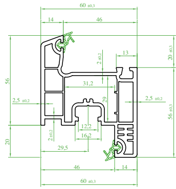
(ST 1310) "GROSSTEC" Kanat Profili (Contalı) Sash Profile (Seal) Профиль створки (с уплотнителем) بروفیل الضرفه (مع القفیل)
