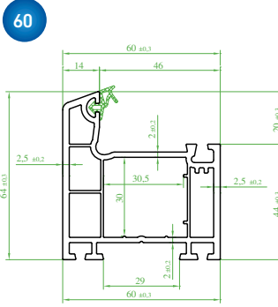
(ST 1110) "GROSSTEC" Kasa Profili (Contalı) Frame Profile (Seal) Профиль коробки (с уплотнителем) بروفیل الصندوق (مع قفیل)
