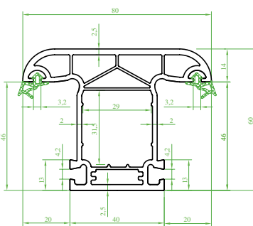
(ST 3210) "OVALTEC" Orta kayıt Profili (Contalı) Mullion profile (Seal) Профиль импоста (с уплотнителем) بروفیل المنصف الثابت (مع القفیل)
