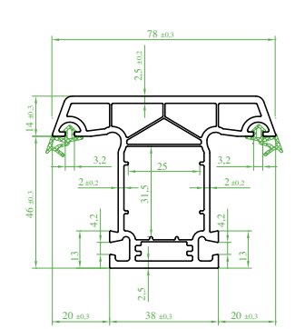
(ST 9210) "EXTRATEC" Orta kayıt Profili (Contalı) Mullion profile (Seal) Профиль импоста (с уплотнителем) بروفیل المنصف الثابت (مع القفیل)
