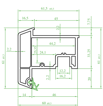
(ST 3310) "OVALTEC" Kanat Profili (Contalı) Sash Profile (Seal) Профиль створки (с уплотнителем) بروفیل الضرفه (مع القفیل)
