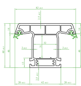
(ST 1210) "GROSSTEC" Orta kayıt Profili (Contalı) Mullion profile (Seal) Профиль импоста (с уплотнителем) بروفیل المنصف الثابت (مع القفیل)
