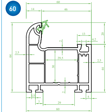
(ST 4110) "SOLOTEC" Kasa Profili (Contalı) Frame Profile (Seal) Профиль коробки (с уплотнителем) بروفیل الصندوق (مع قفیل)
