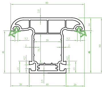
(ST 4210) "SOLOTEC" Orta kayıt Profili (Contalı) Mullion profile (Seal) Профиль импоста (с уплотнителем) بروفیل المنصف الثابت (مع القفیل)
